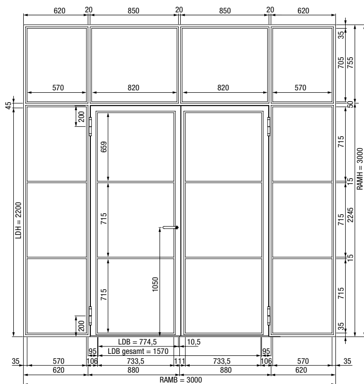
2-flügelige Drehflügeltür mit Seitenteilen und Oberlicht
