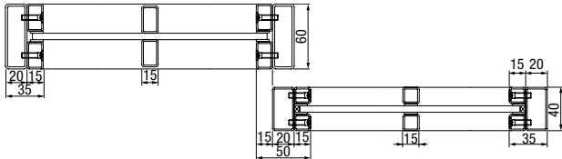
Horizontalschnitt
