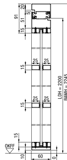
Vertikalschnitt
