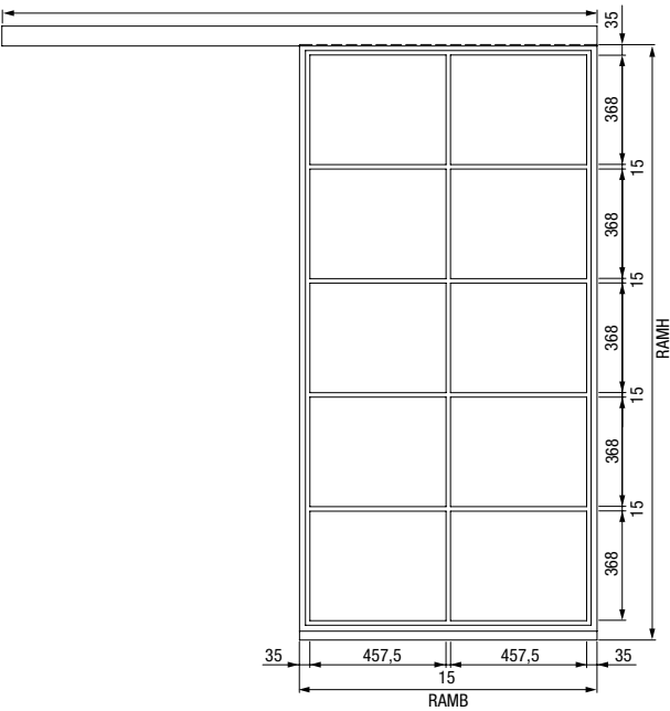
1-flüglige Schiebetür
