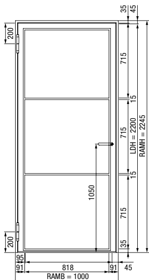
1-flügelige Drehflügeltür
