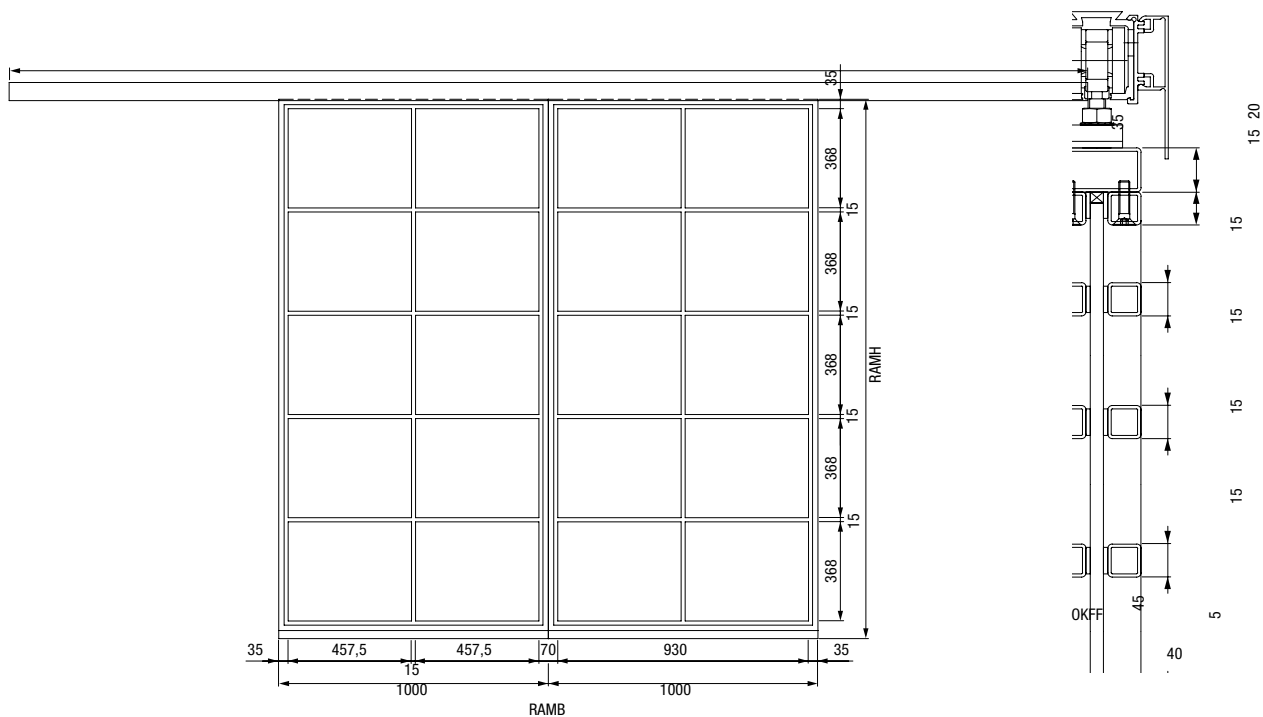
1-flüglige Schiebetür
