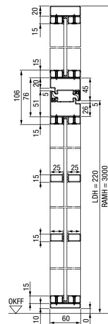
Vertikalschnitt
