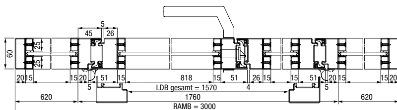
Horizontalschnitt
