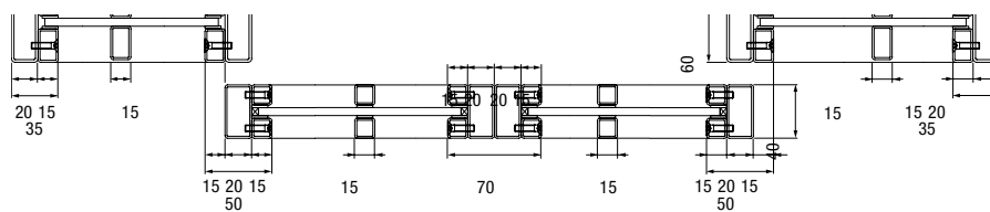
Horizontalschnitt
