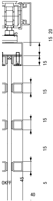
Vertikalschnitt
