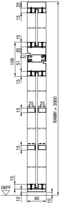
Vertikalschnitt
