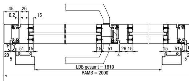
Horizontalschnitt 2-flügelige Drehflügeltür
