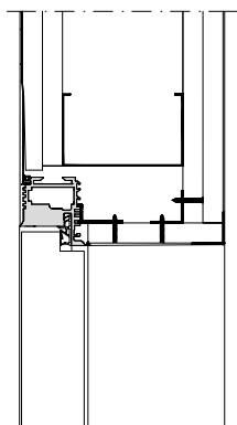
Vertikalschnitt normal nach außen öffnend (Typ NA)
