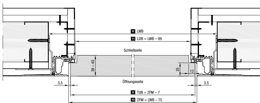
Horizontalschnitt Typ NA mit normal öffnendem Türblatt
