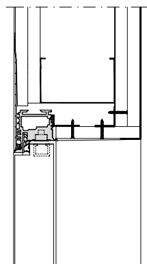
Vertikalschnitt revers in die Türleibung öffnend (Typ RI)
