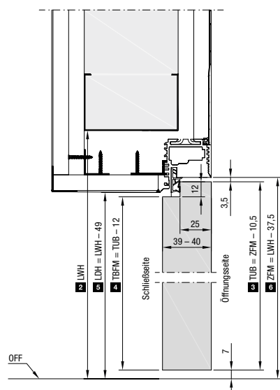
Vertikalschnitt Typ NA mit normal öffnendem Türblatt
