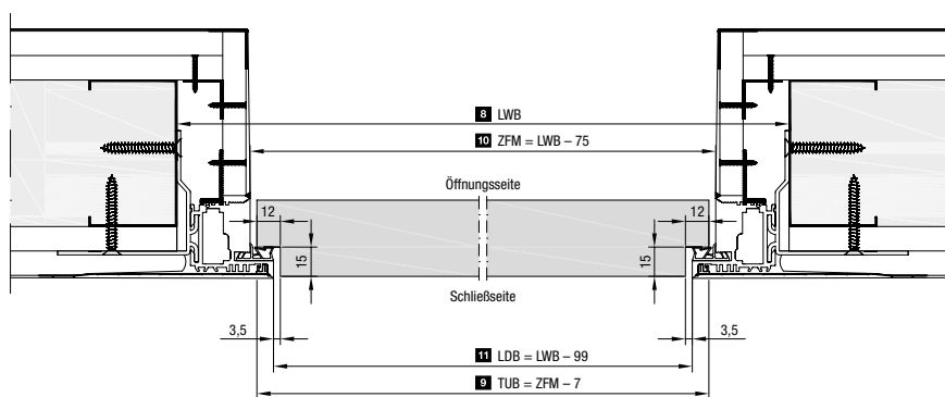
Horizontalschnitt Typ RI mit revers öffnendem Türblatt
