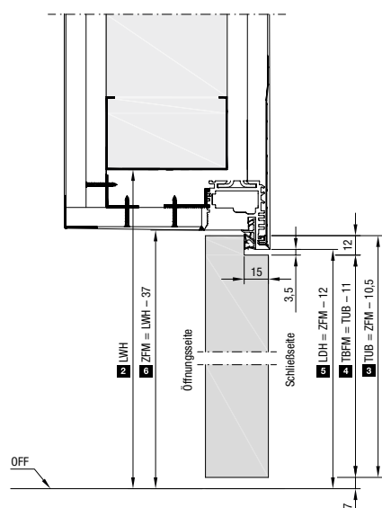
Vertikalschnitt Typ RI mit revers öffnendem Türblatt
